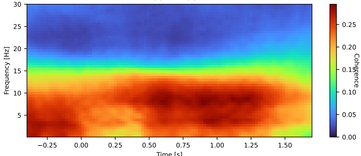
8B (2) - dPFC (5)
